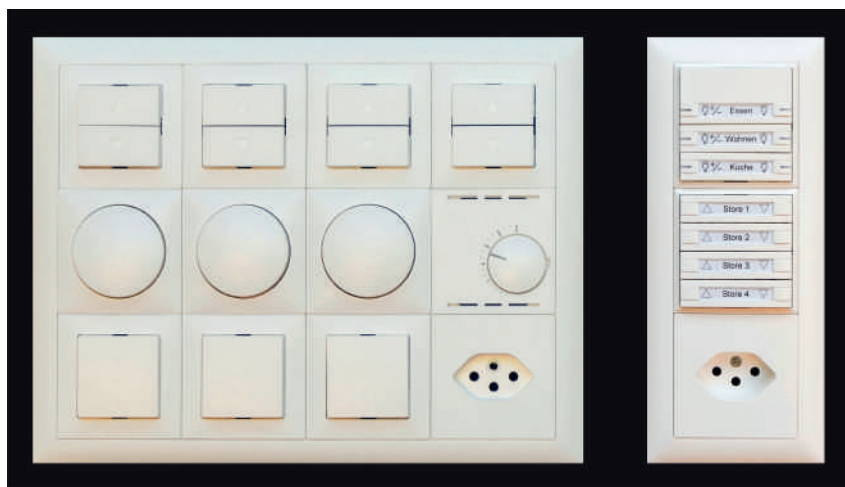
Der Unterschied auf einen Blick: Links: Eine konventionelle «Taster-Batterie» für 4 Storen, 3 Dimmer und 3 Lichter. Rechts: Mit NOXnet genügt ein Viertel des Platzes für alle Funktionen, inklusive Thermostat für Einzelraumregulierung.
